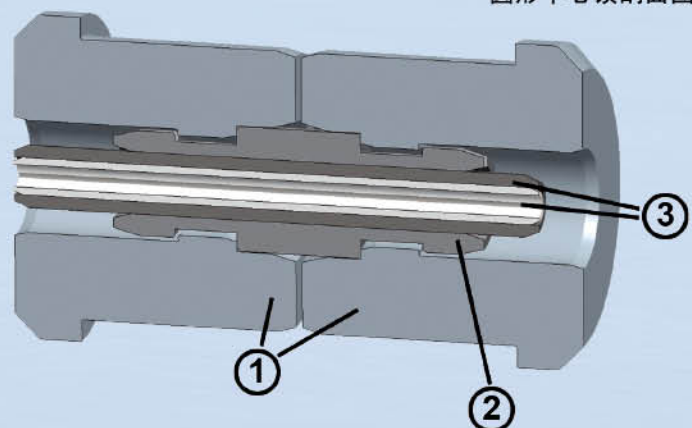
圆形中间锁剖面图
