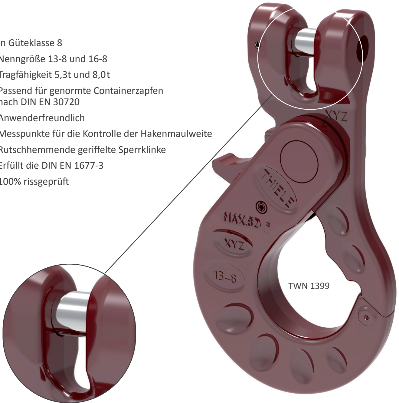
mit Ovalbolzen
